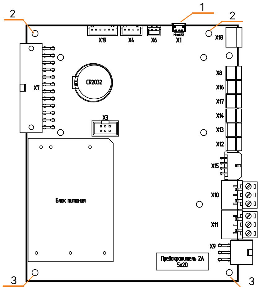
Рис.13 Плата контроллера
